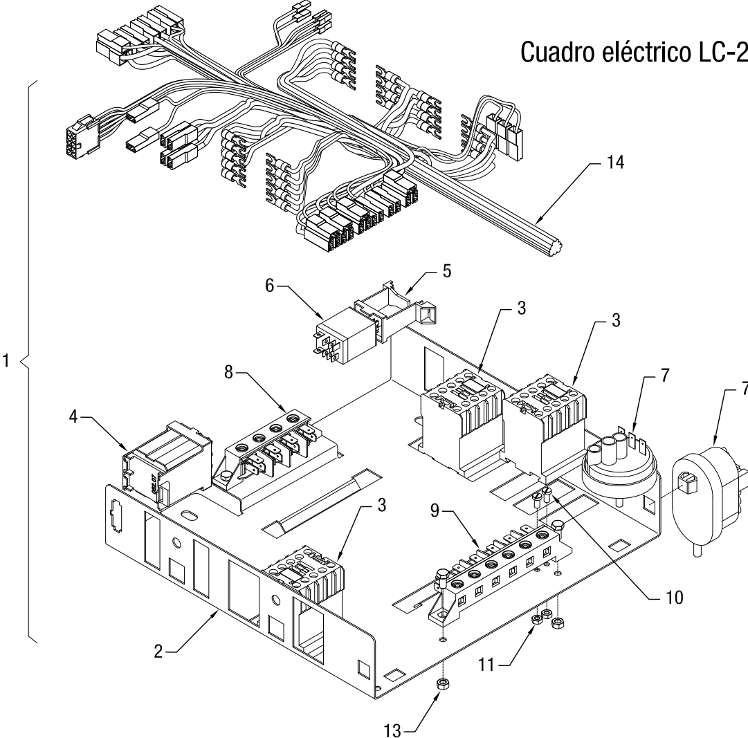
Cuadro eléctrico LC-2800 // LC-2300TR-230V 3~
