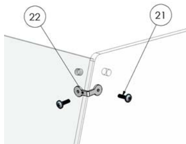
DETALLE ESCUADRA MONTAJE CRISTAL .
